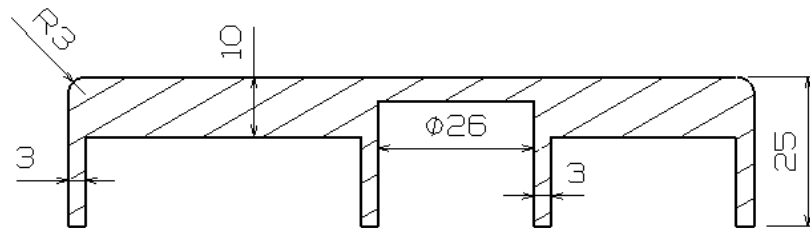
Section cut A-A Scale: 1:1
