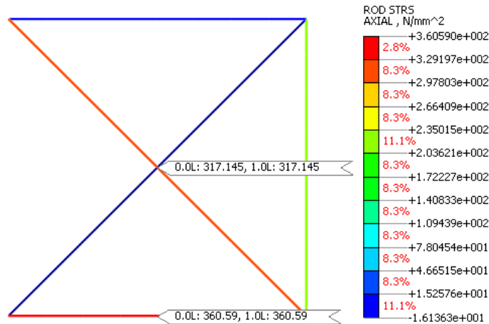
응력 결과
