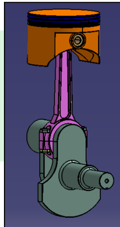
조립체 모델
