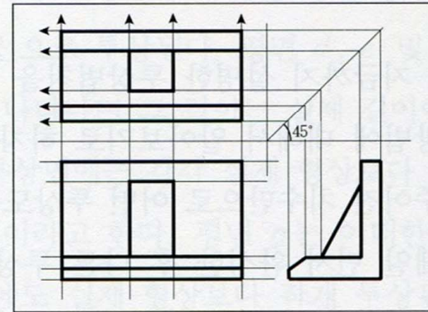
(4) 평면도를 완성한다.
