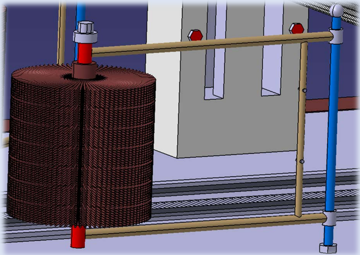
측면 Brush
