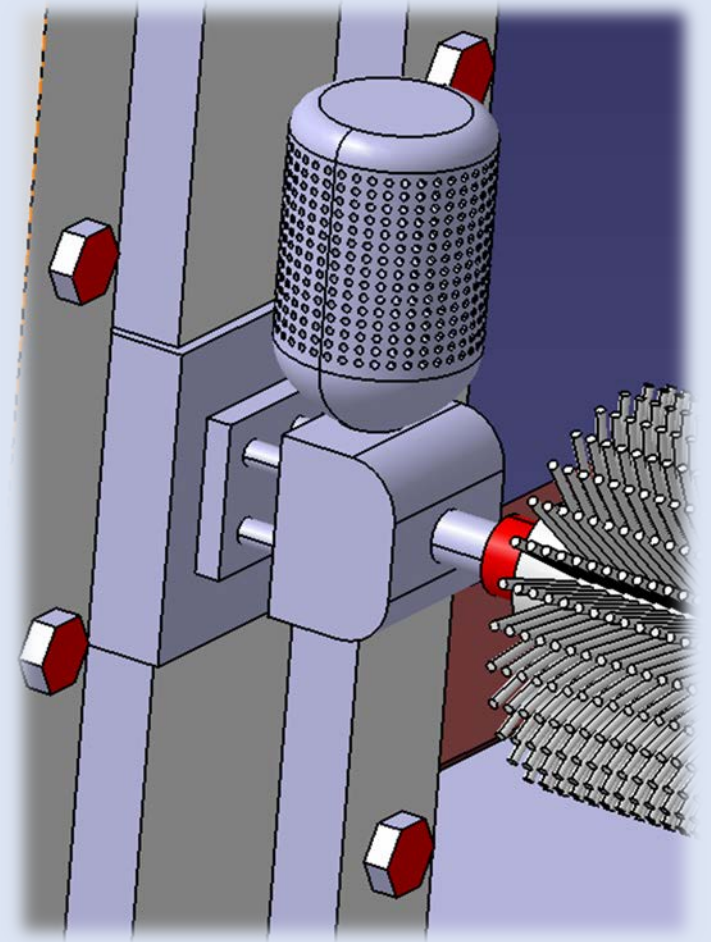
Brush 구동부
