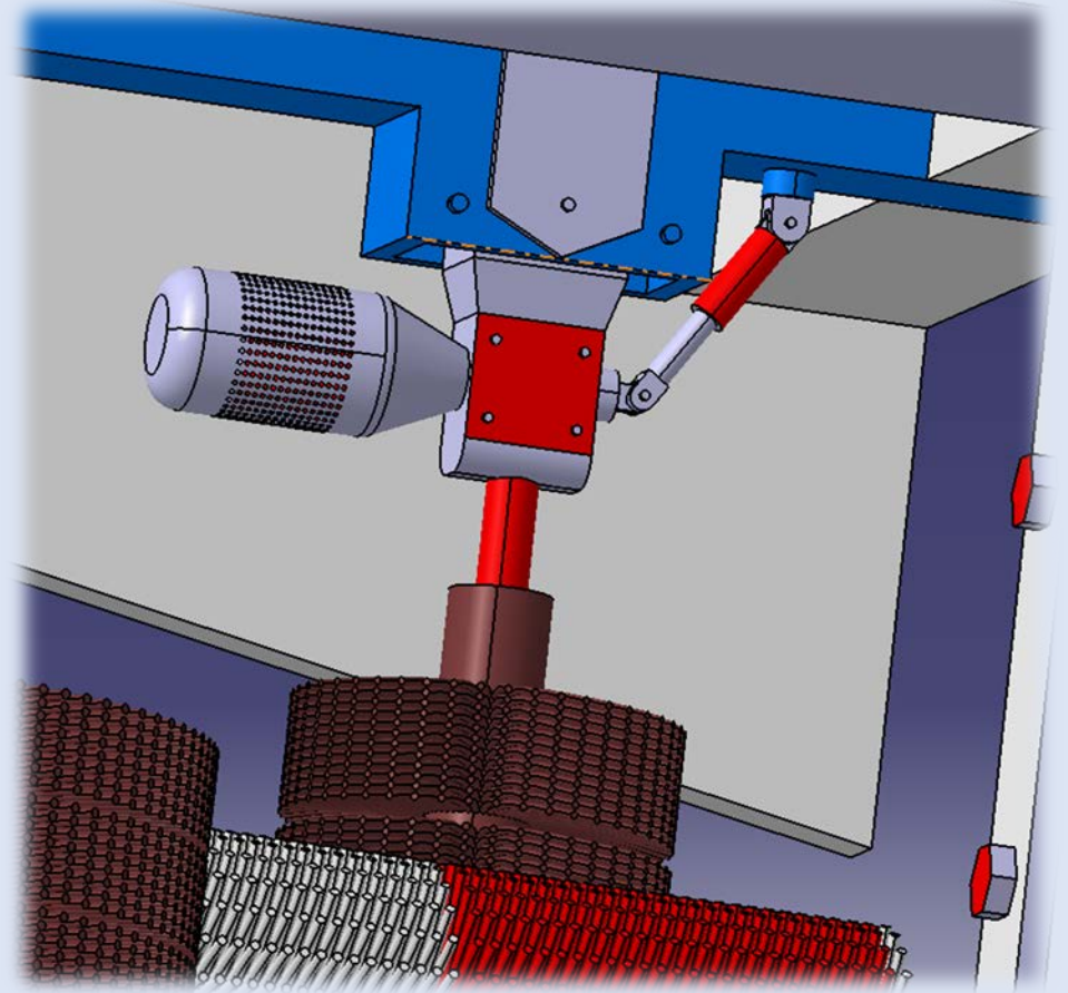
Brush 구동부
